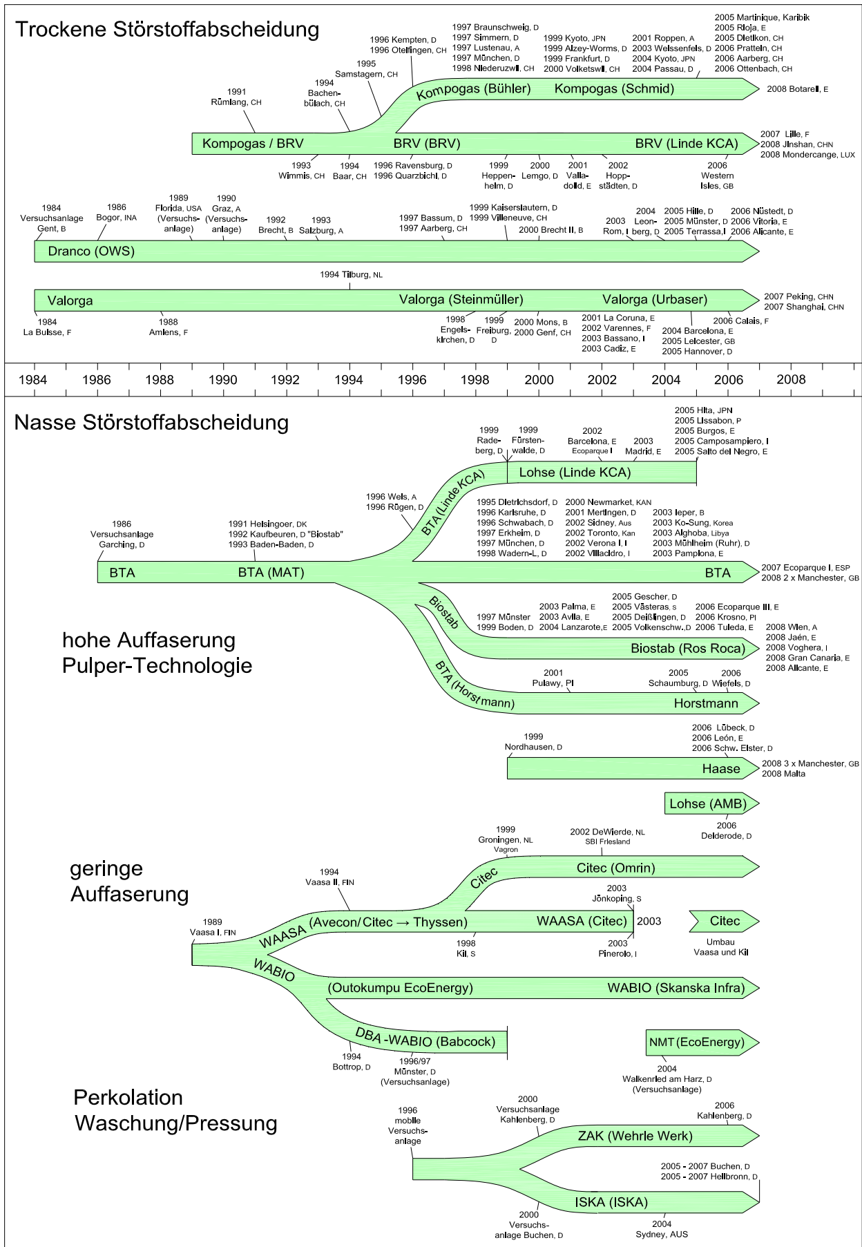
Abbildung 1: Entwicklung der Vergärungsverfahren
