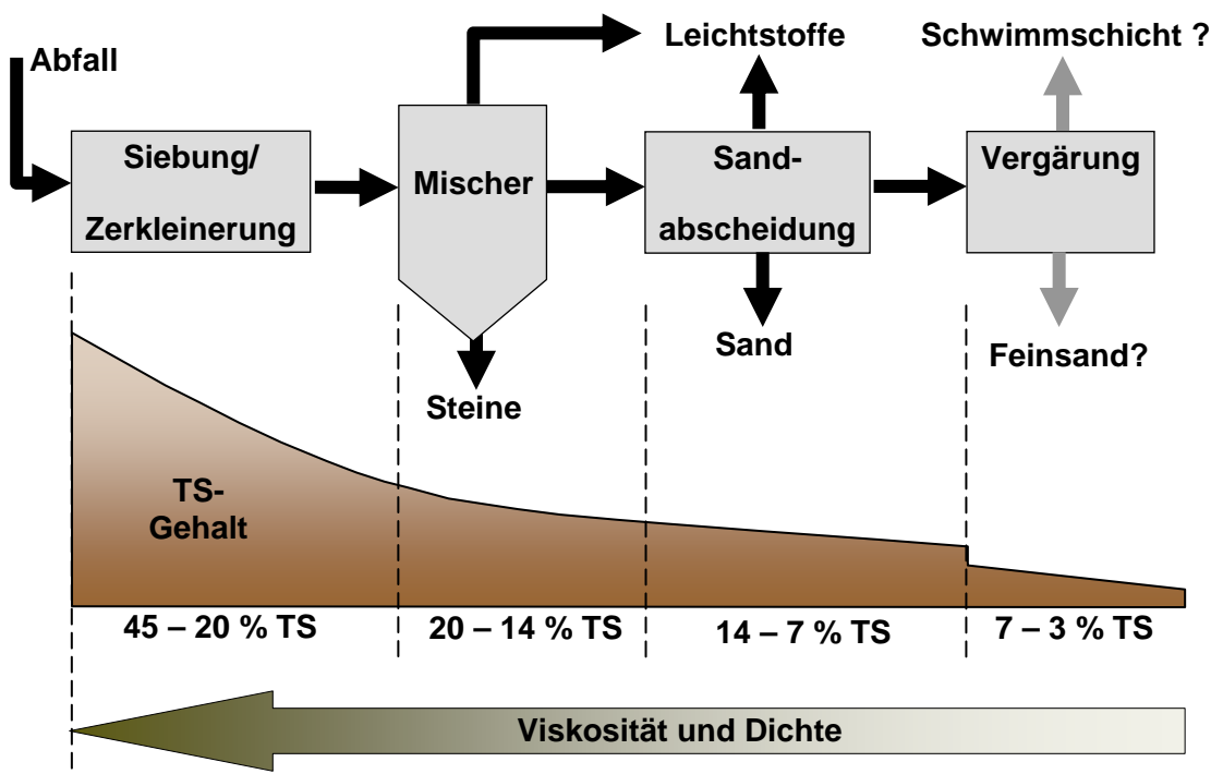
Abbildung 2: Prinzipien der Störstoffabscheidung bei der Nassvergärung
